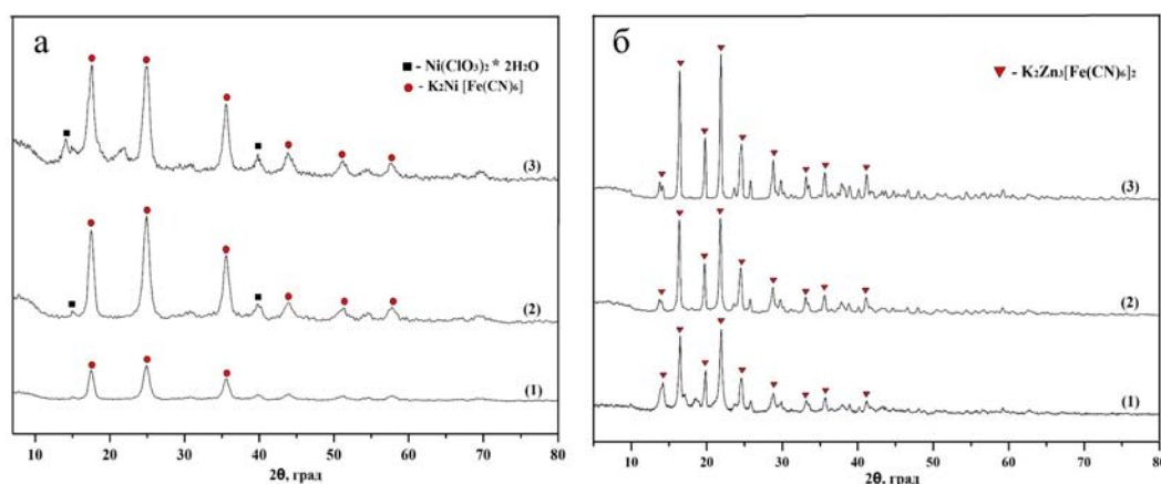
Рис. 1. Рентгенограммы полученных образцов: а) (1) – FC K-Ni; (2) – FC K-Ni-PE, (3) – FC K-Ni PE-Em; б) (1) – FC K-Zn; (2) – FC K-Zn-PE, (3) – FC K-Zn-PE-Em
