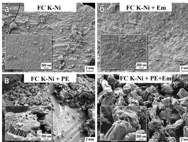
Рис. 2. РЭМ изображения поверхности смешанных ФЦ K-Ni: (а) – исходный, (б) – добавлением силиоксан-акрилатной эмульсии, (в) – с добавлением полиэтилена, (г) – с добавлением полиэтилена и силиоксан-акрилатной эмульсии
