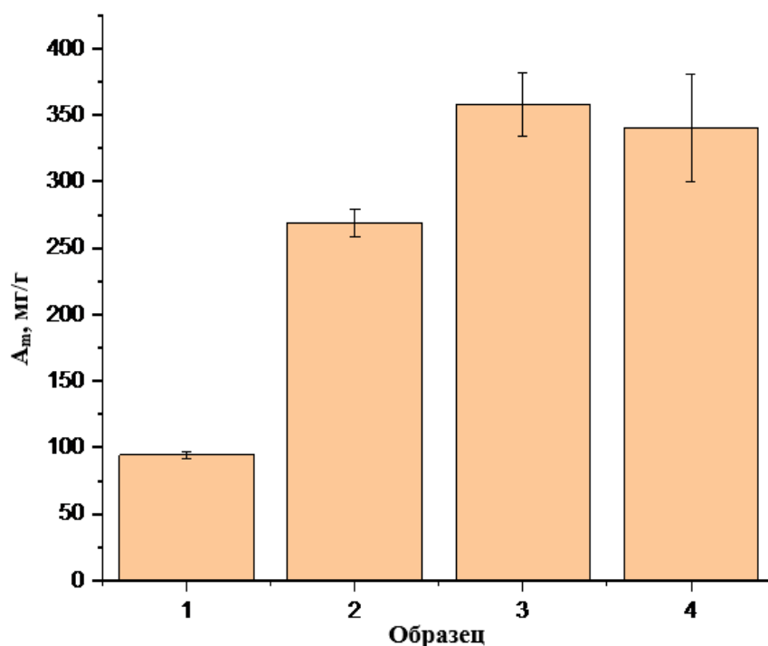
Рис. 3. Значения максимальной сорбционной емкости образцов алюмосиликатов с соотношением Si/Al: 1 – 1, 2 – 1.5, 3 – 2.0, 4 – 2.5
