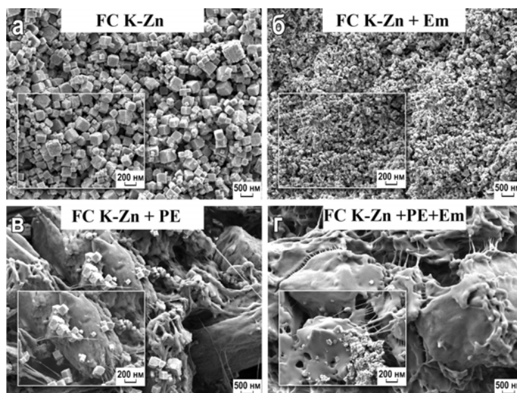
Рис. 3. РЭМ изображения поверхности смешанных ФЦ K-Zn: (а) – исходный, (б) – с добавлением силиоксан-акрилатной эмульсии, (в) – с добавлением полиэтилена, (г) – с добавлением полиэтилена и силиоксан-акрилатной эмульсии
