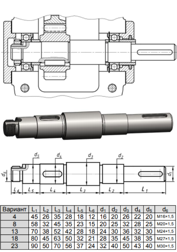
Материал вала – Сталь 40Х ГОСТ 4543-2016
