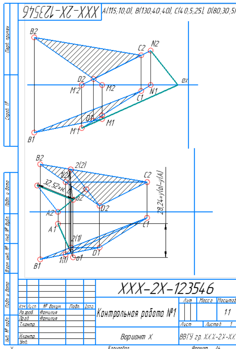
Рисунок 5.2.2 — Определение расстояния от точки А до плоскости
