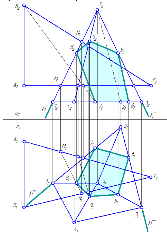
Рисунок 5.2.4 – Построение сечения
