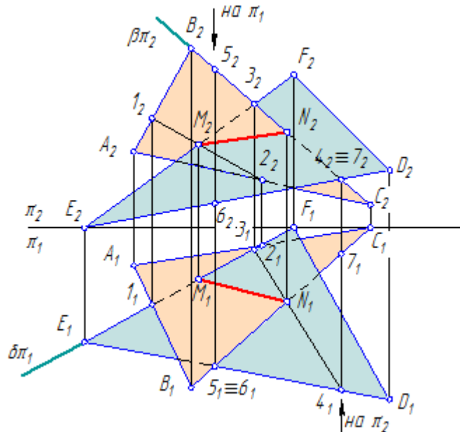
Рисунок 5.2.3 – Построение линии пересечения двух плоскостей
