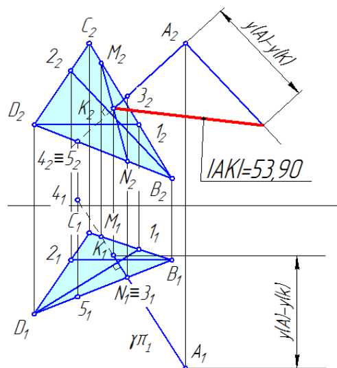
Рисунок 5.2.2 — Определение расстояния от точки А до плоскости
