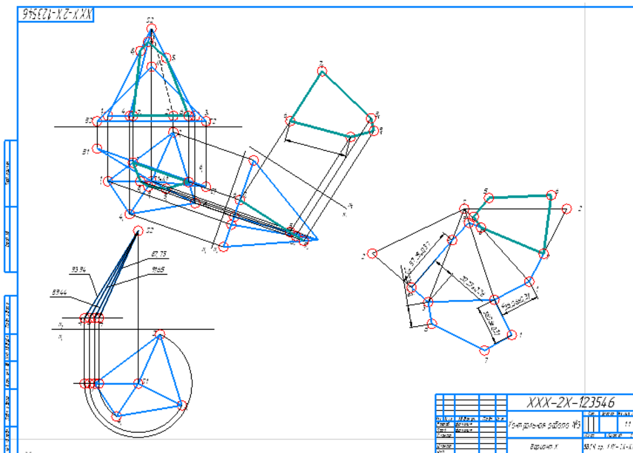
Рисунок 5.2.5 – Пересечение пирамиды плоскостью общего положения
