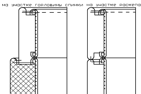
Рисунок 11. Схема метода поузловой обработки и соединения с горловиной обтачного отложного воротника (припуск шва обтачивания настроен на нижний воротник) и соединение с горловиной изделий пальтово-костюмного ассортимента плечевой группы
