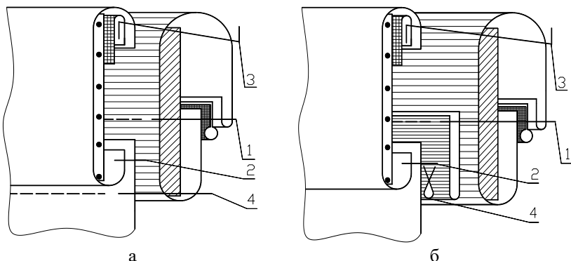
Рисунок 23. Схемы методов технологической обработки верхнего среза мужских брюк
