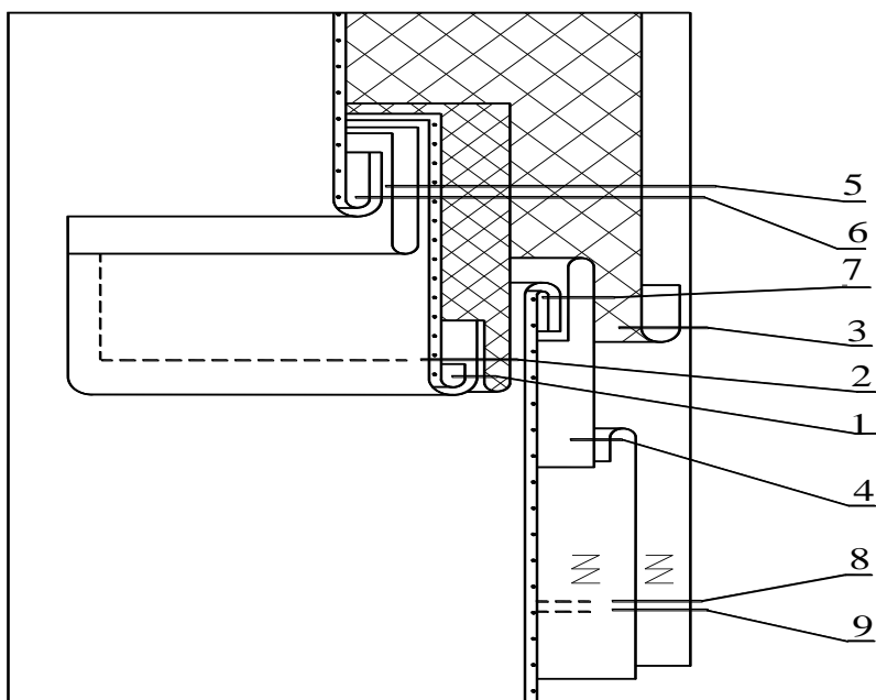
Рисунок 8. Схема метода технологической обработки бокового прорезного кармана с клапаном и двумя обтачками
