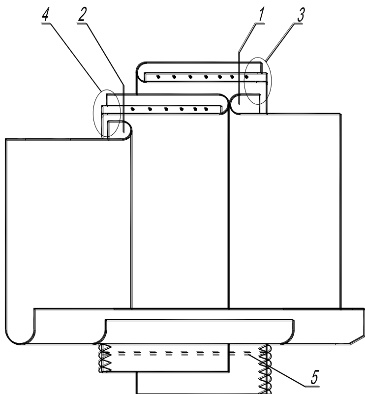
Рисунок 27. Схема технологической обработки застежки втачными планками в изделиях платьево-блуточного ассортимента с застежкой до верха
