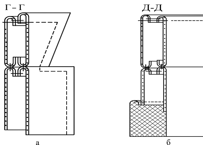
Рисунок 13. Схема метода технологической обработки отложного воротника и соединение его с горловиной жакета с отложными лацканами: а) на участке горловины спинки; б) на участке раскепа
