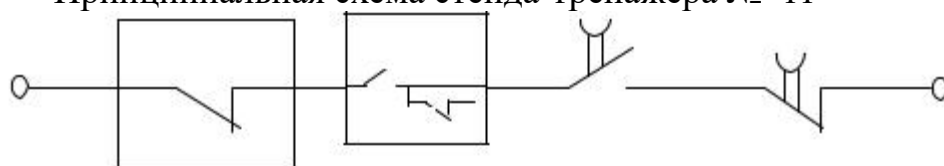
Принципиальная схема стенда-тренажера № 11
