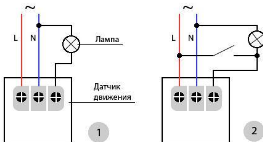
Принципиальная схема стенда-тренажера № 14
