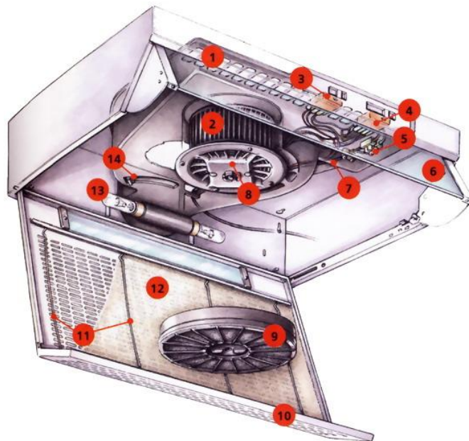
Рис. 2 Рециркуляционная вытяжка
