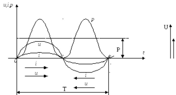
Рис. 3. Волновые и векторные диаграммы резистивного элемента
