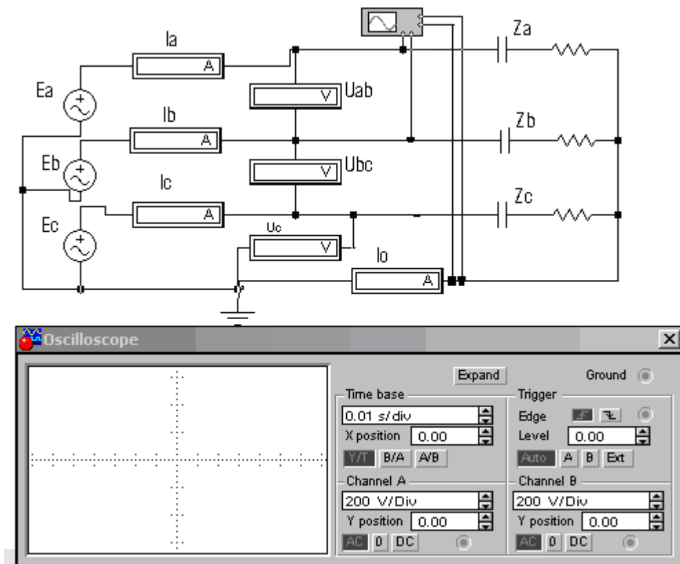
Рис. 3.Схема моделирования системы звезда-звезда с симметричной нагрузкой (осциллограф измеряет фазное и линейное напряжения)
