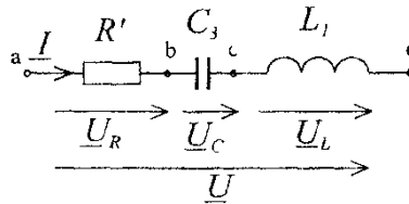
Рис.1. Схема последовательного соединения элементов
