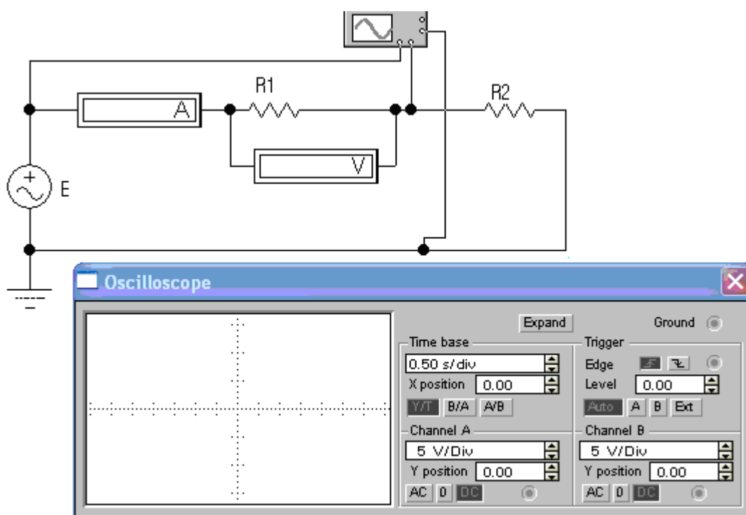
Рис. 4. Экспериментальная схема
