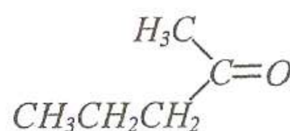
метилпропилкетон
