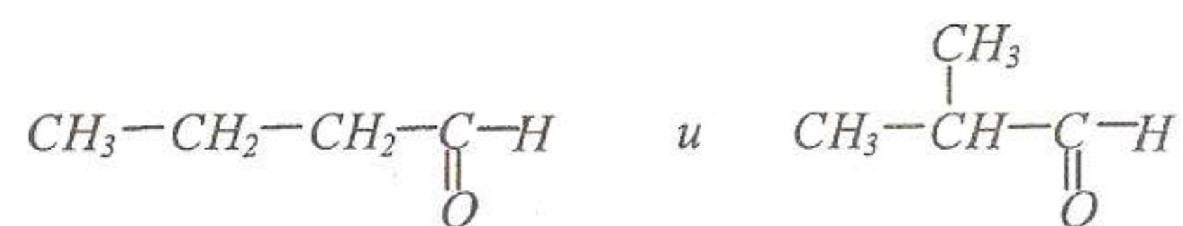
масляный альдегид
