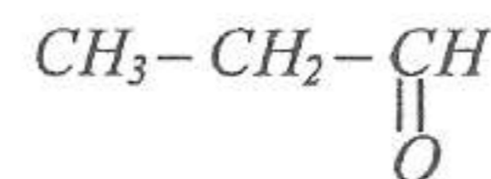
пропиловый альдегид
