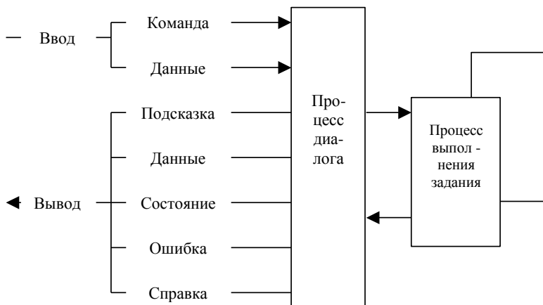
Рис. 41. Типы сообщений диалога
