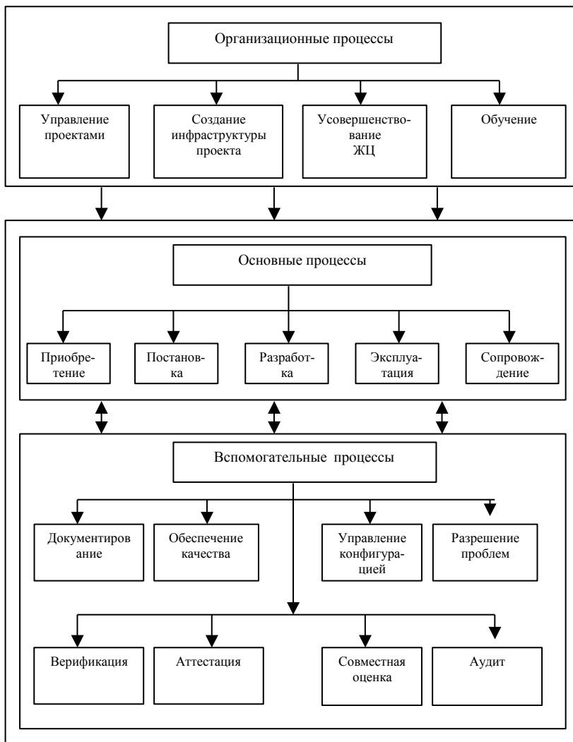
Рис. 5. Процессы ЖЦ ПО
