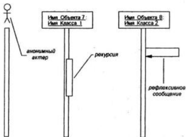
Рис. 33. Графическое изображение актера, рекурсии и рефлексивного сообщения
