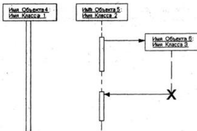
Рис. 32. Графическое изображение различных вариантов линий жизни и фокусов управления объектов
