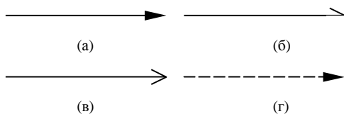
Рис. 34. Графическое изображение различных видов сообщений между объектами на диаграмме последовательности
