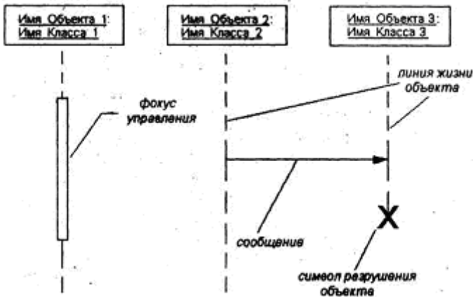
Рис. 31. Различные графические примитивы диаграммы последовательности
