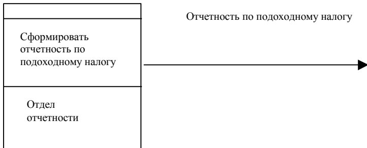
Рис. 19. Поток данных
