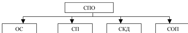
Рис. 2. Классификация СПО
