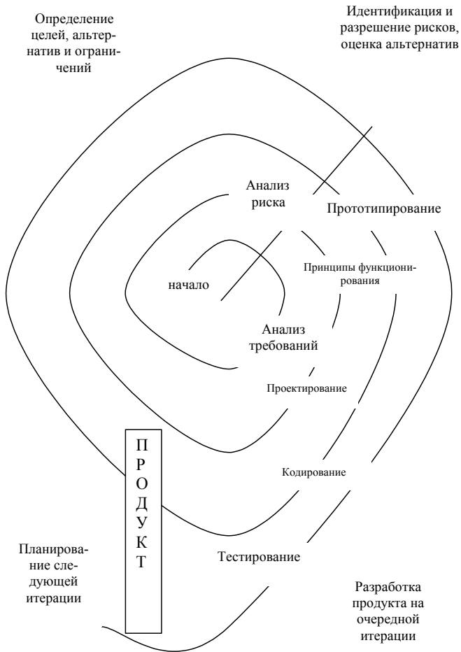
Рис. 8. Спиральная модель
