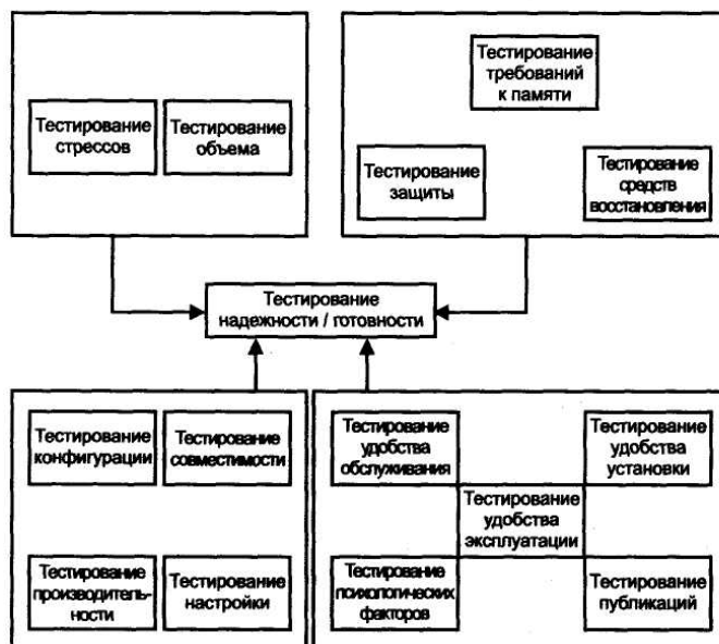
Рис. 44. Схема проектирования комплексного теста
