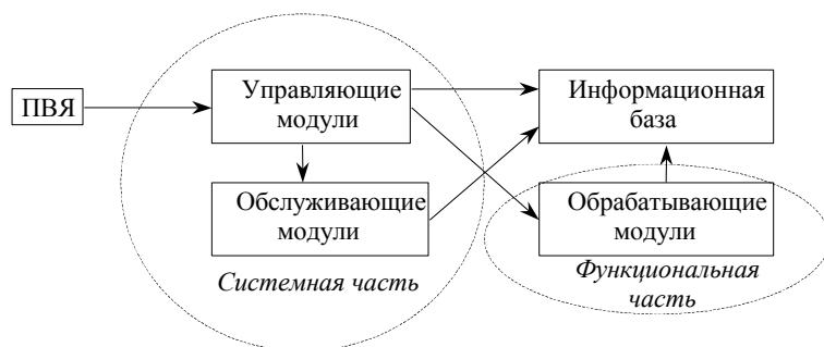
Рис. 4. Классификация СПО
