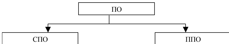
Рис. 1. Классификация ПО
