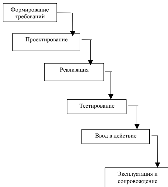
Рис. 6. Каскадная схема разработки ПО
