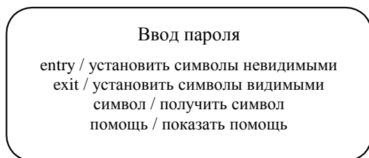
Рис. 36. Пример состояния с непустой секцией внутренних действий
